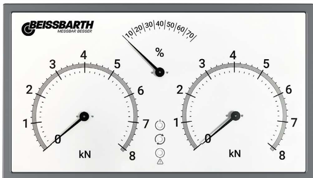
Analoganzeige Analoganzeige mit Wandhalterung, Bestellnummer: 1 691 401 100
